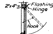
SECTION D-D
