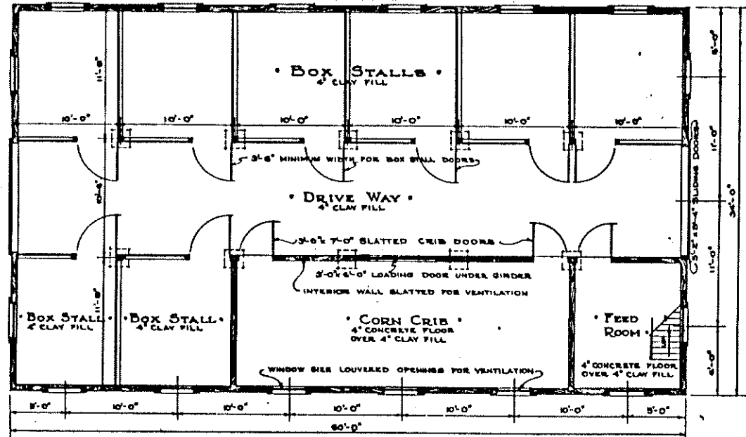
• FLOOR PLAN •
