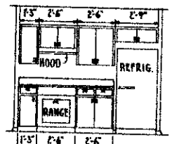
ELEVATION B
