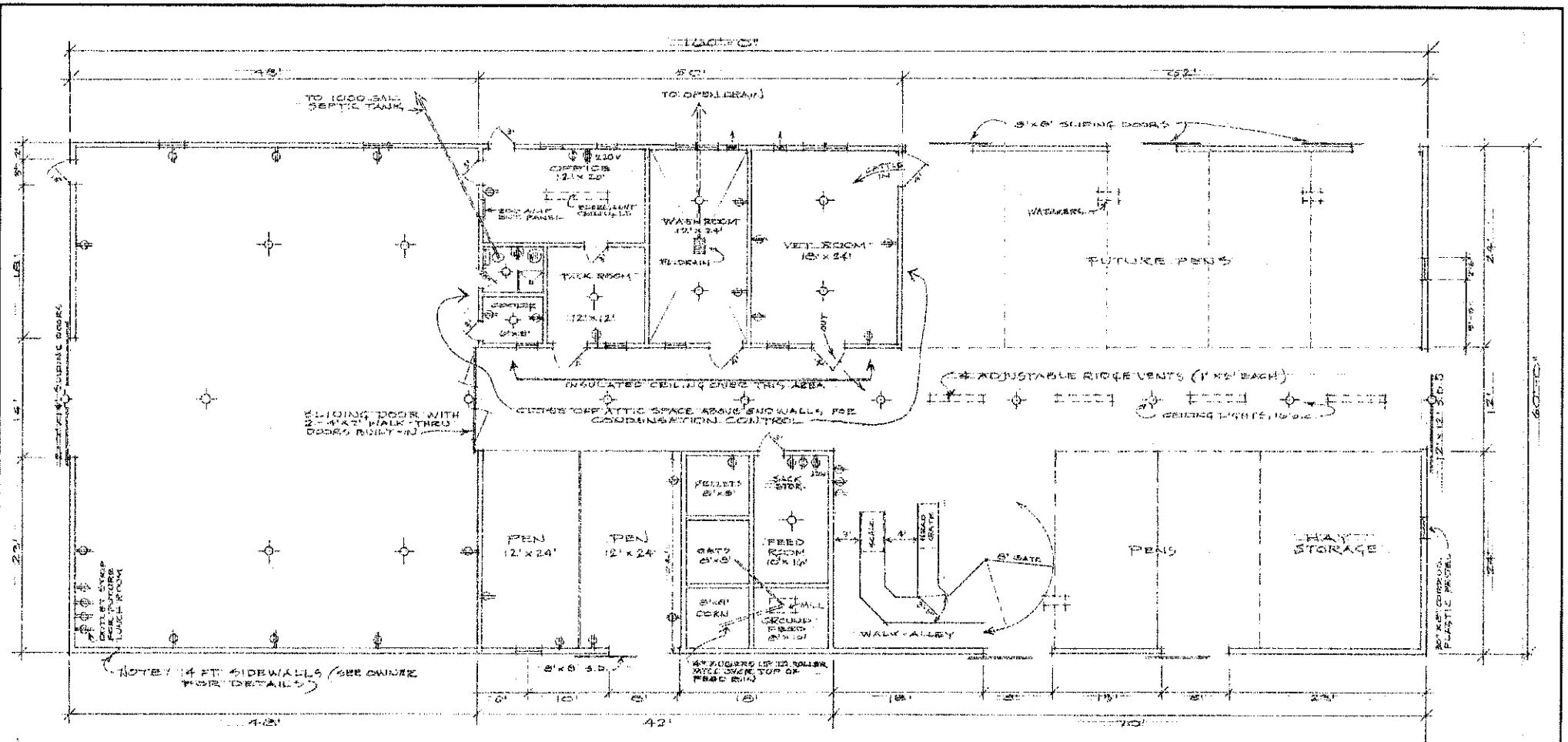
FLOOR PLAN SCALE: 1/8" = 1'-0"
