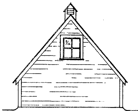
BACK VIEW SCALE: \frac{3}{8} = 1'-0"
