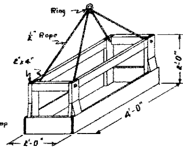
DUMB WAITER Scale: \frac{1}{2} " = 1'-0"
