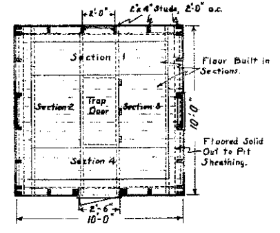
FLOOR PLAN Scale: \frac{1}{4} " = 1'-0"
