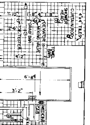
SECTION D-D
