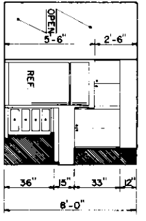
ELEV. 1
