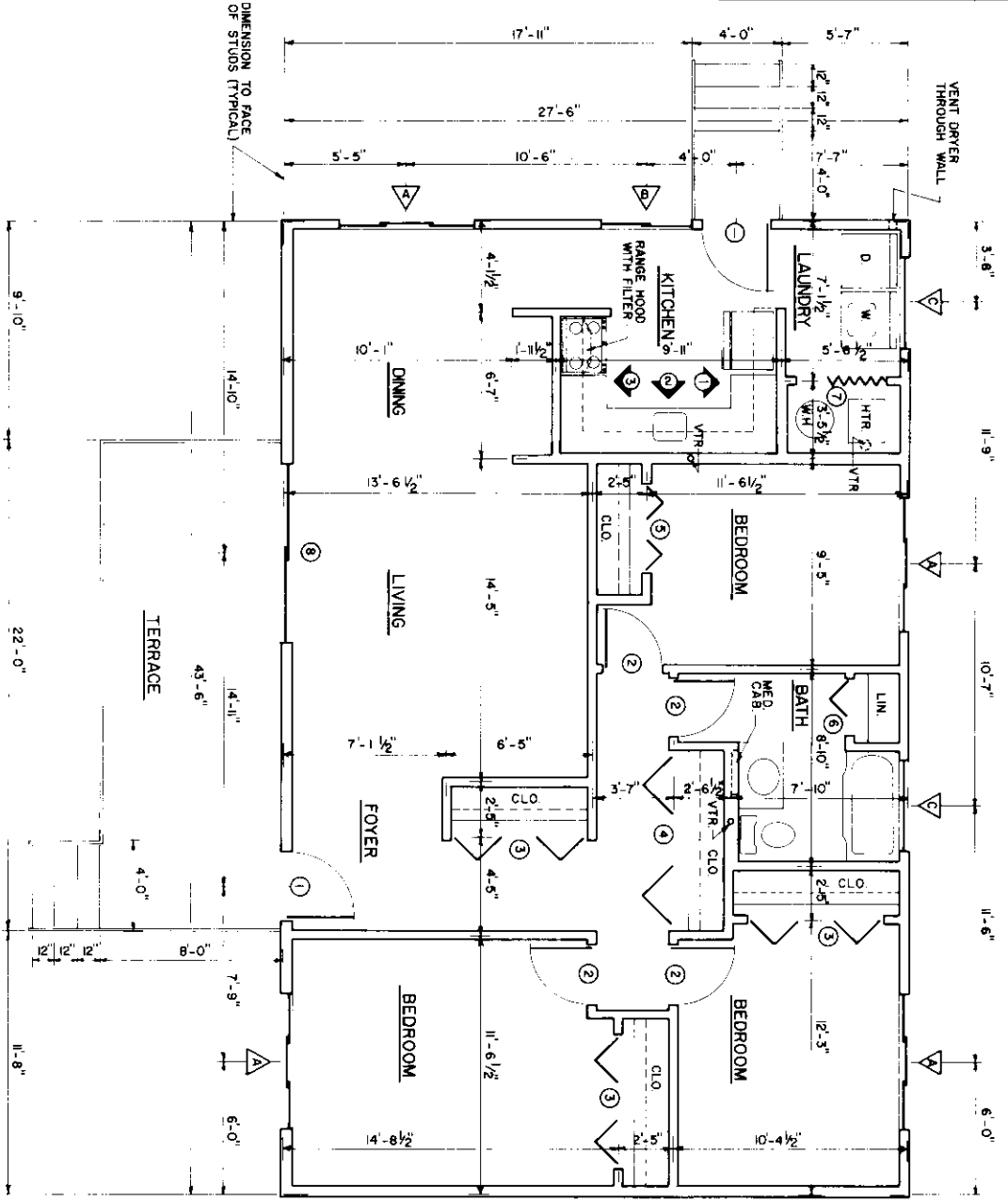
PLAN SCALE: 1/4" = 1'-0"
