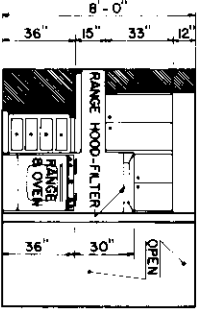
ELEV. 3
