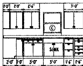
ELEVATION A
