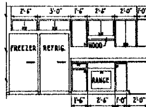
ELEVATION B
