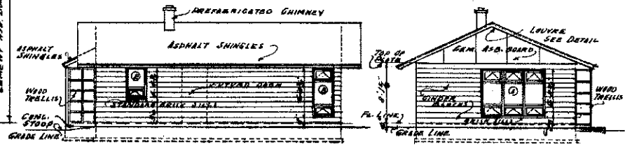
ELEVATION -C' ELEVATION -D'
