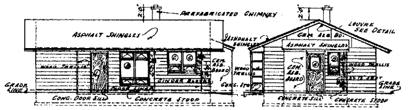
ELEVATION -A' ELEVATION -B'
