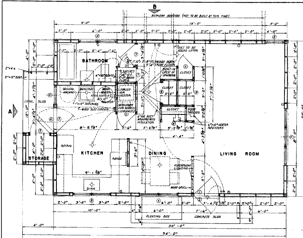
FLOOR PLAN SCALE: 3/8" = 1'-0"
