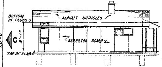
ELEVATION B
