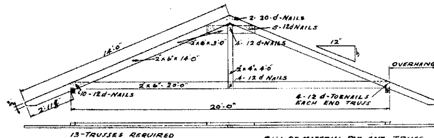
TRUSS DETAIL SCALE: 3/8" = 1'-0"
