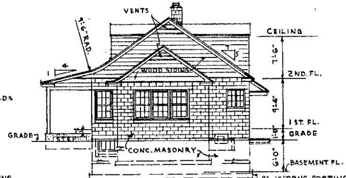
RIGHT ELEVATION
