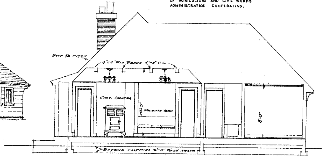
• LONGITUDINAL SECTION •
