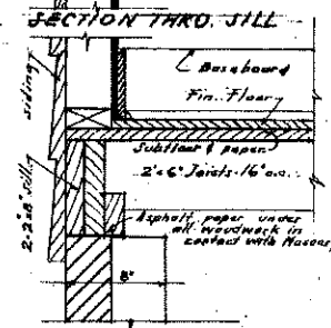
SECTION THRO SILL Scale: 1/8" = 1'-0"
