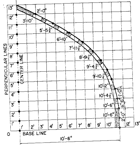
VPI & SU GOTHIC RAFTER SCALE: 1/2" = 1'-0"
