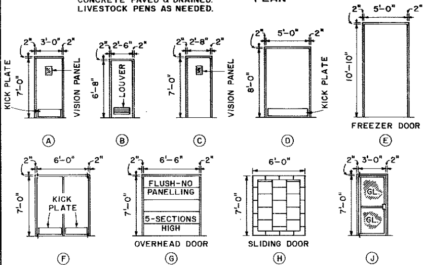
DOOR SCHEDULE
