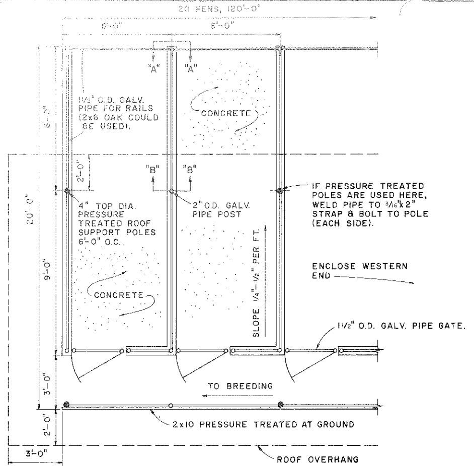
PLAN SCALE: 3/8"=1'-0"
