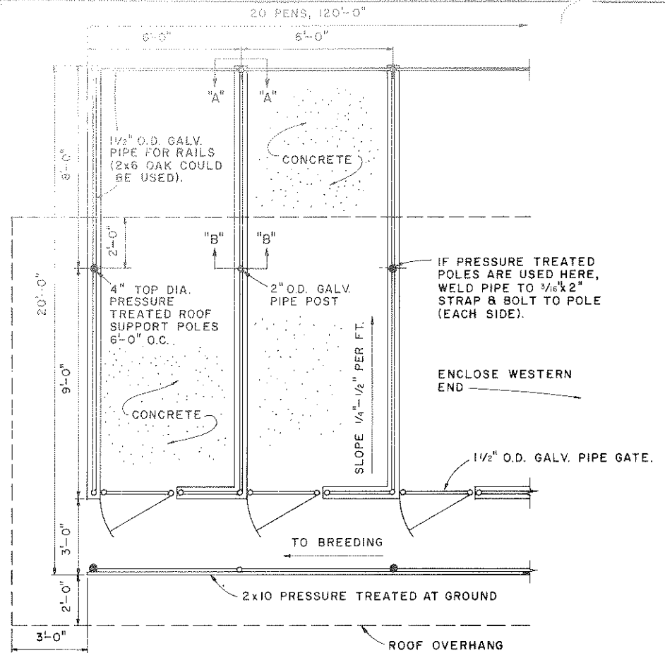
PLAN SCALE: 3/8"=1'-0"
