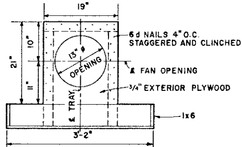
END ELEVATION
