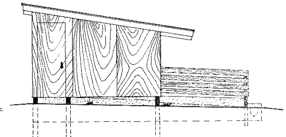
END ELEVATION
