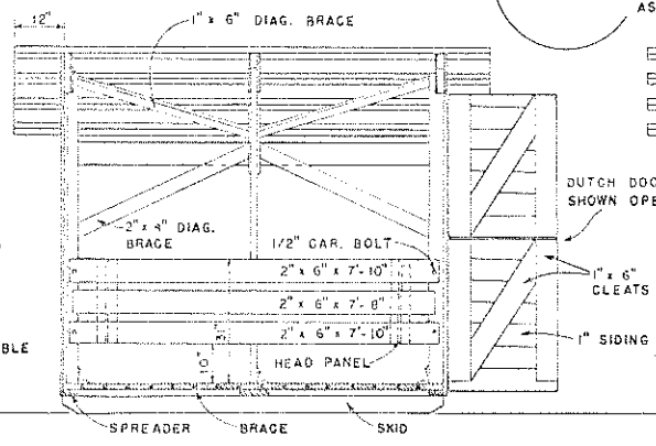
LONGITUDINAL SECTION
