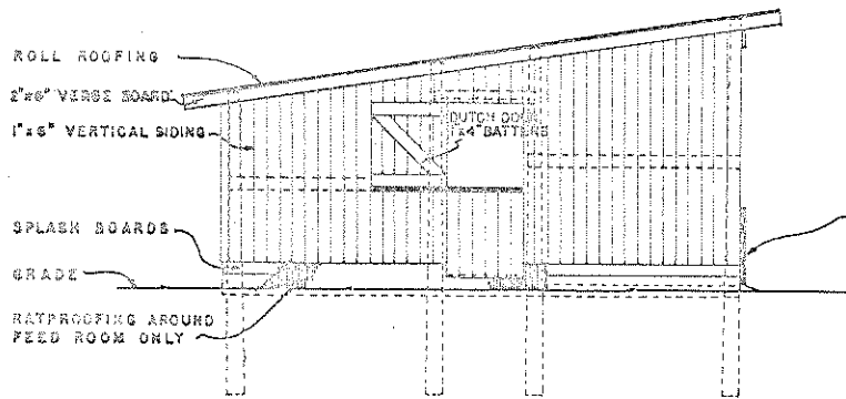
END ELEVATION
