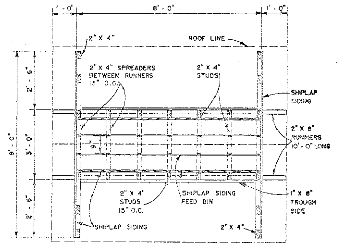
PLAN A-A
