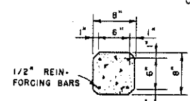
SECTION A-A SCALE: 0 1 2 3 4 FT.
