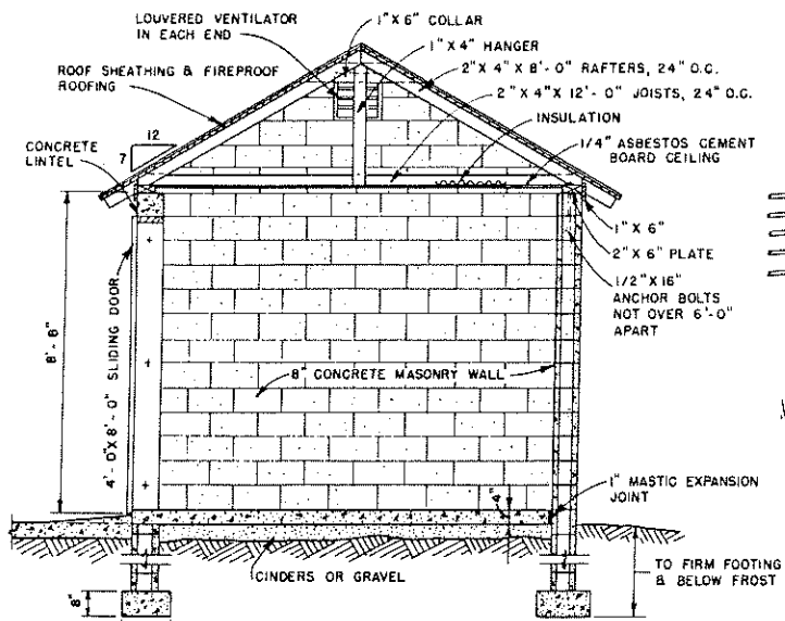
SECTION A-A SCALE: 0 1 2 3 4 FT.
