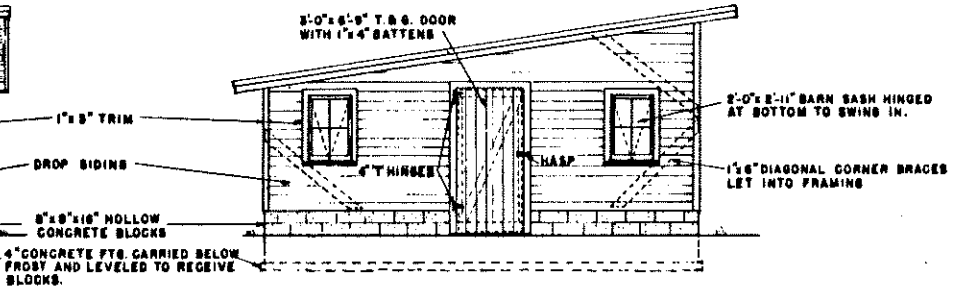
END ELEVATION
