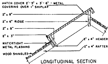
LONGITUDINAL SECTION
