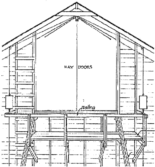
HAY DOOR SERVICE PLATFORM
