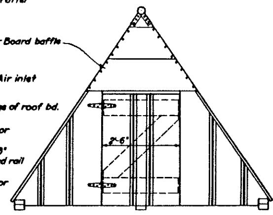
END ELEVATION
