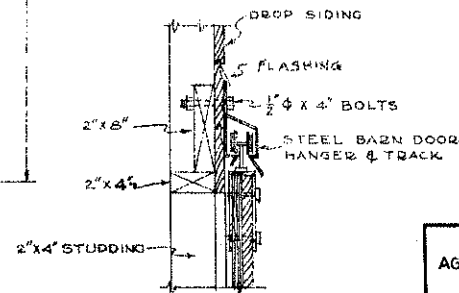
SLIDING DOOR DETAILS
