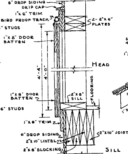
HAY MOW DOOR SCALE \frac{1}{2}'' = 1'-0''
