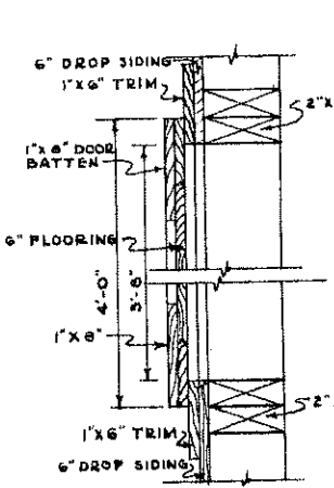
JAMB
