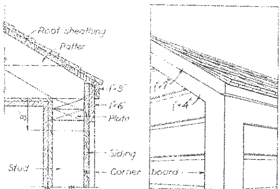
CORNICE NO-3
