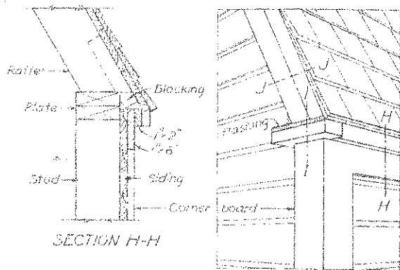
CORNICE NO-1
