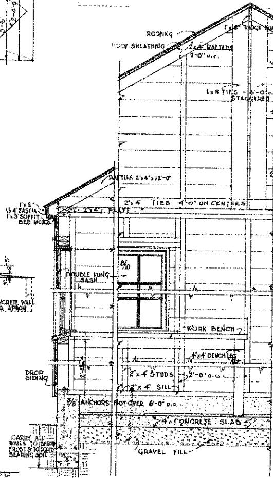
SECTION A-A
